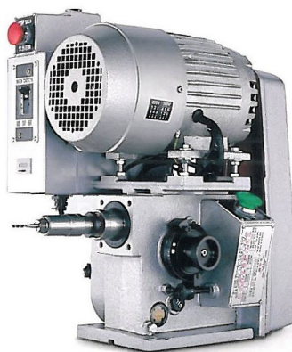
MTM-08H Horizontal Fully Automatic Tapping Machine 臥式全自動攻牙機
